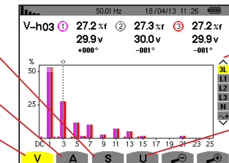
Obrázek 51: Obrazovka režimu harmonických
