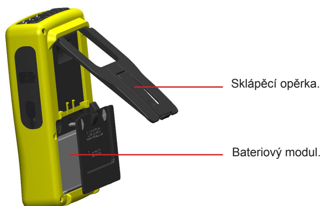
Obrázek 5: Opěrka a krytka přihrádky pro bateriový modul
