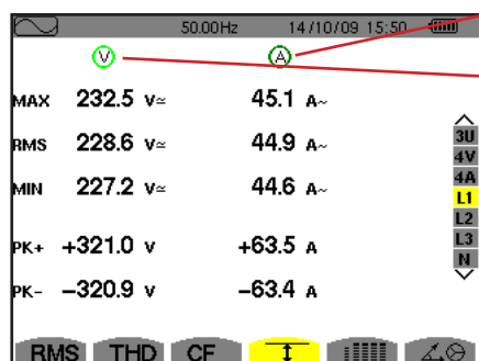
Obrázek 76: Obrazovka L1 Max.-Min.
