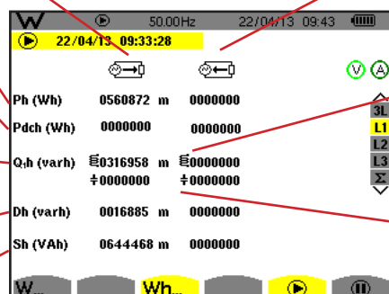
Obrázek 114: Obrazovka spotřebovaných a generovaných energií v L1
