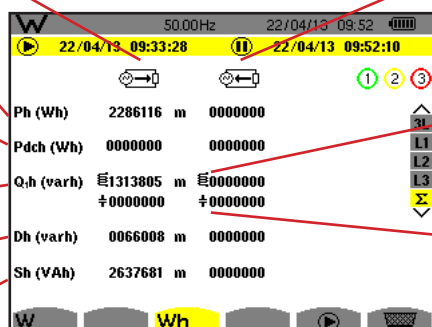
Obrázek 116: Obrazovka celkových energií spotřebovaných a generovaných v Σ
