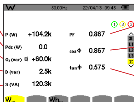
Obrázek 115: Obrazovka celkových výkonů a přiřazených veličin v \Sigma
