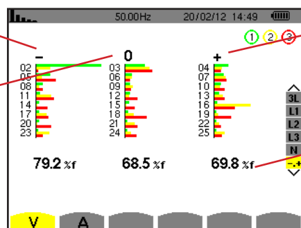
Obrázek 60: Obrazovka expertního režimu napětí mezi fází a nulovým vodičem (třífázové soustavy s nulovým vodičem)
