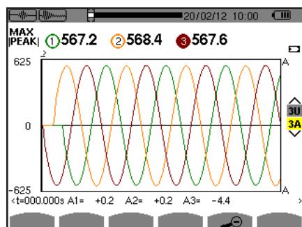
Obrázek 49: Obrazovka 3A PEAK pro 3vodičové třífázové zapojení
