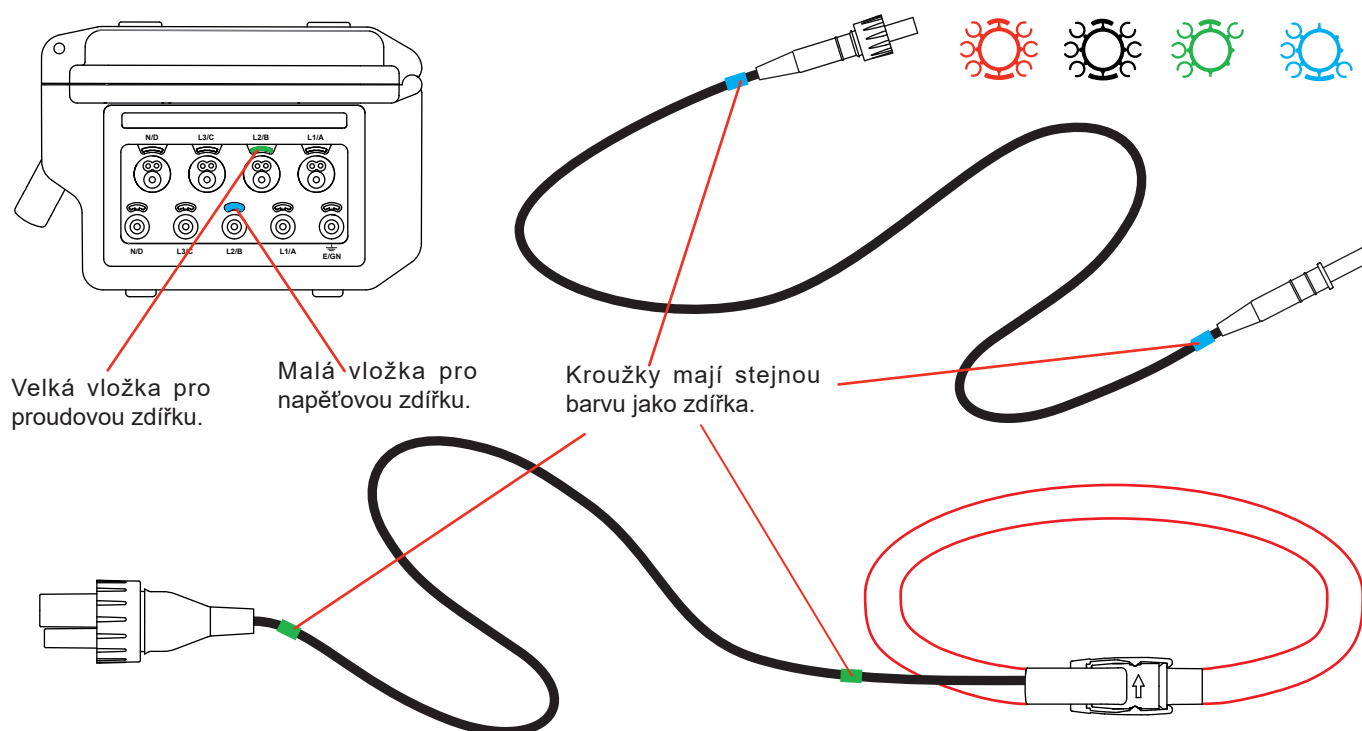
Obrázek 8: značení kabelů
