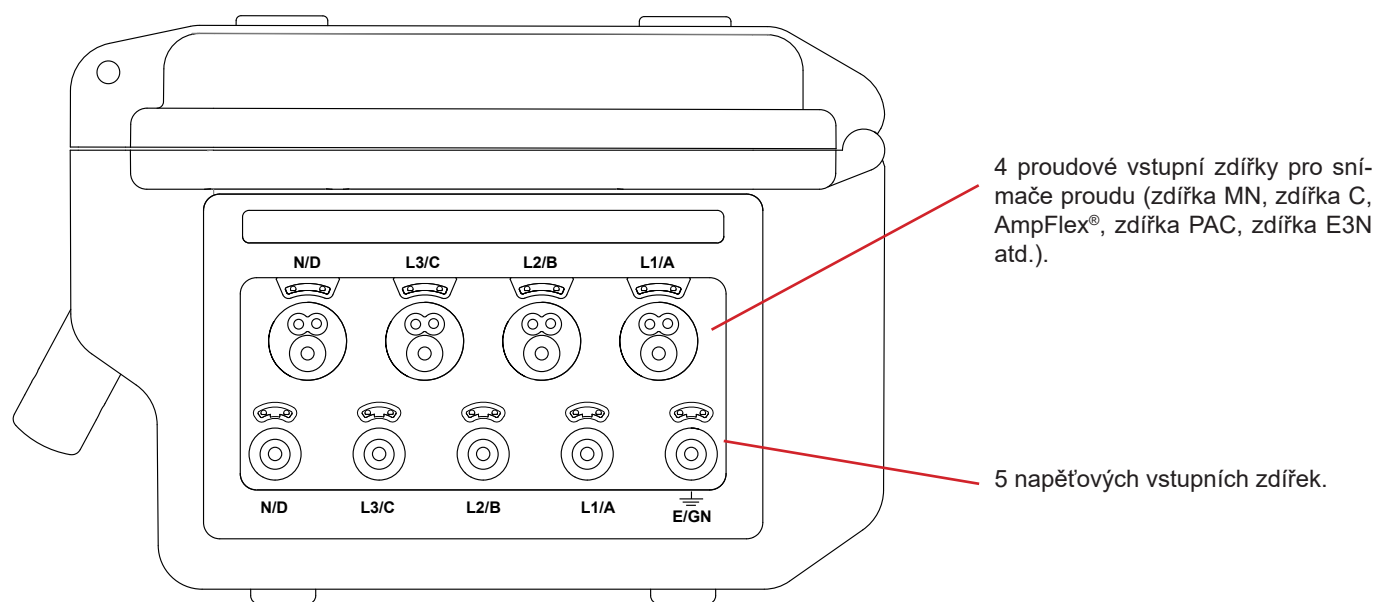
Obrázek 3: Připojovací zdířky
