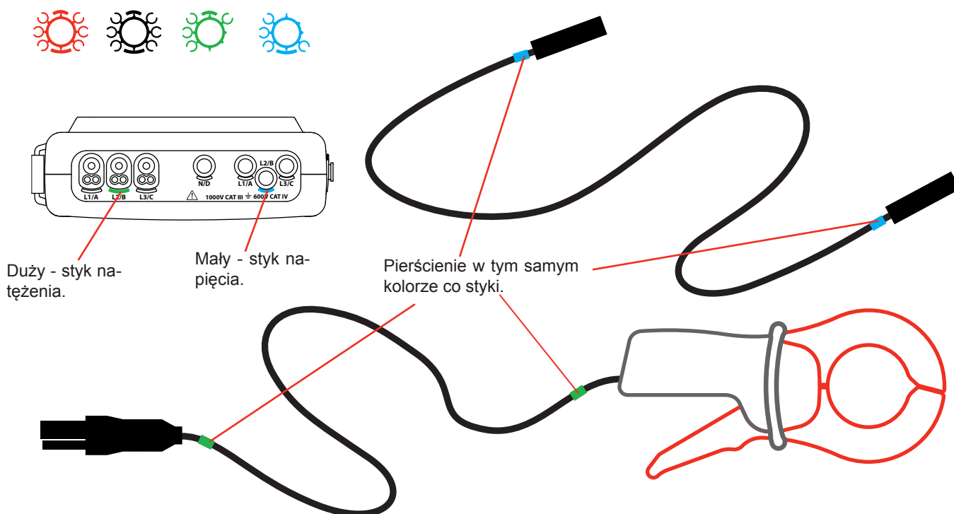
Rysunek 10 : Identyfikacja przewodów i styków
