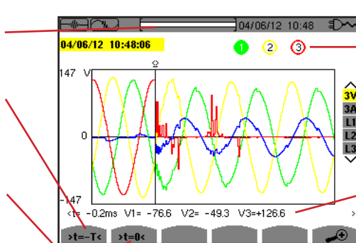
Rysunek 40 : Przykład wyświetlania stanów przejściowych w postaci wykresów dla podłączenia trójfazowego z 4 przewodami
