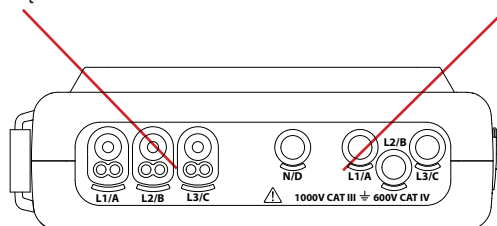
Rysunek 11 : Styki podłączeniowe
