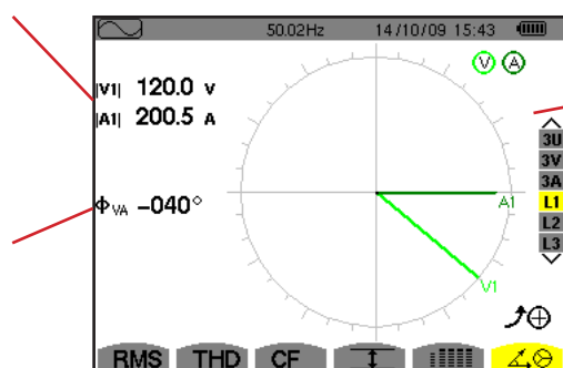
Rysunek 72 : Ekran wyświetlania wykresu Fresnela w L1
