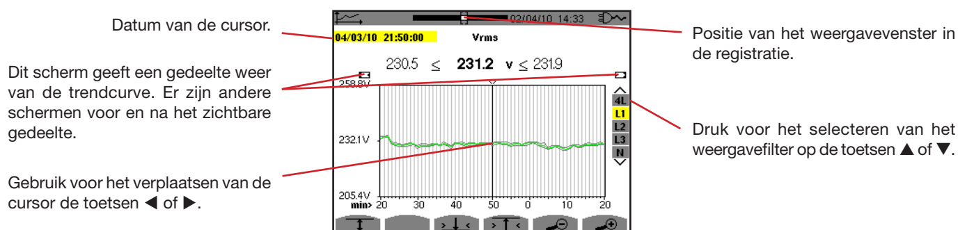
Figuur 95: Vrms (L1) zonder MIN-AVG-MAX
