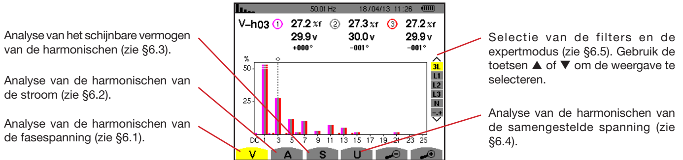
Figuur 51 : het scherm van de harmonische modus
