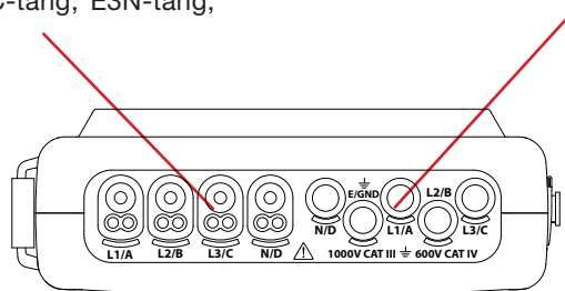
Figuur 3 : de aansluitklemmen
