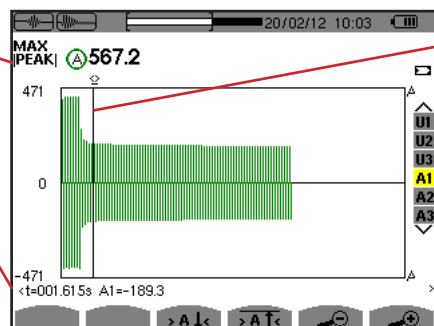
Figuur 50 : het beeldscherm PEAK in A1 voor een driefasen aansluiting zonder nulleider
