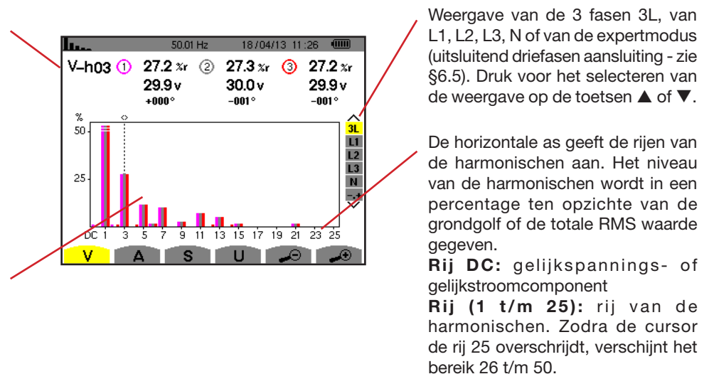
Figuur 52 : voorbeeld van de weergave van de harmonischen van de fasespanning in 3L
