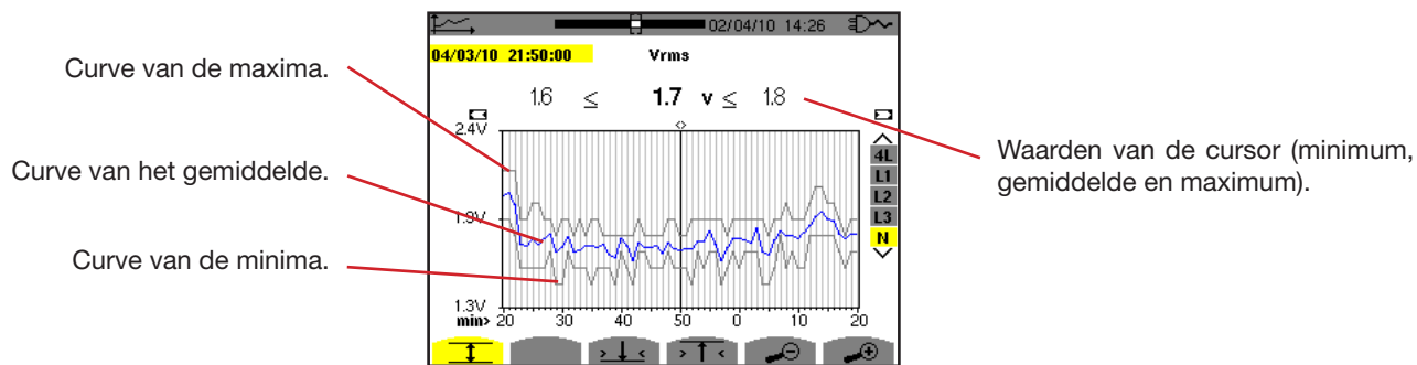
Figuur 94: Vrms (N) met MIN-AVG-MAX
