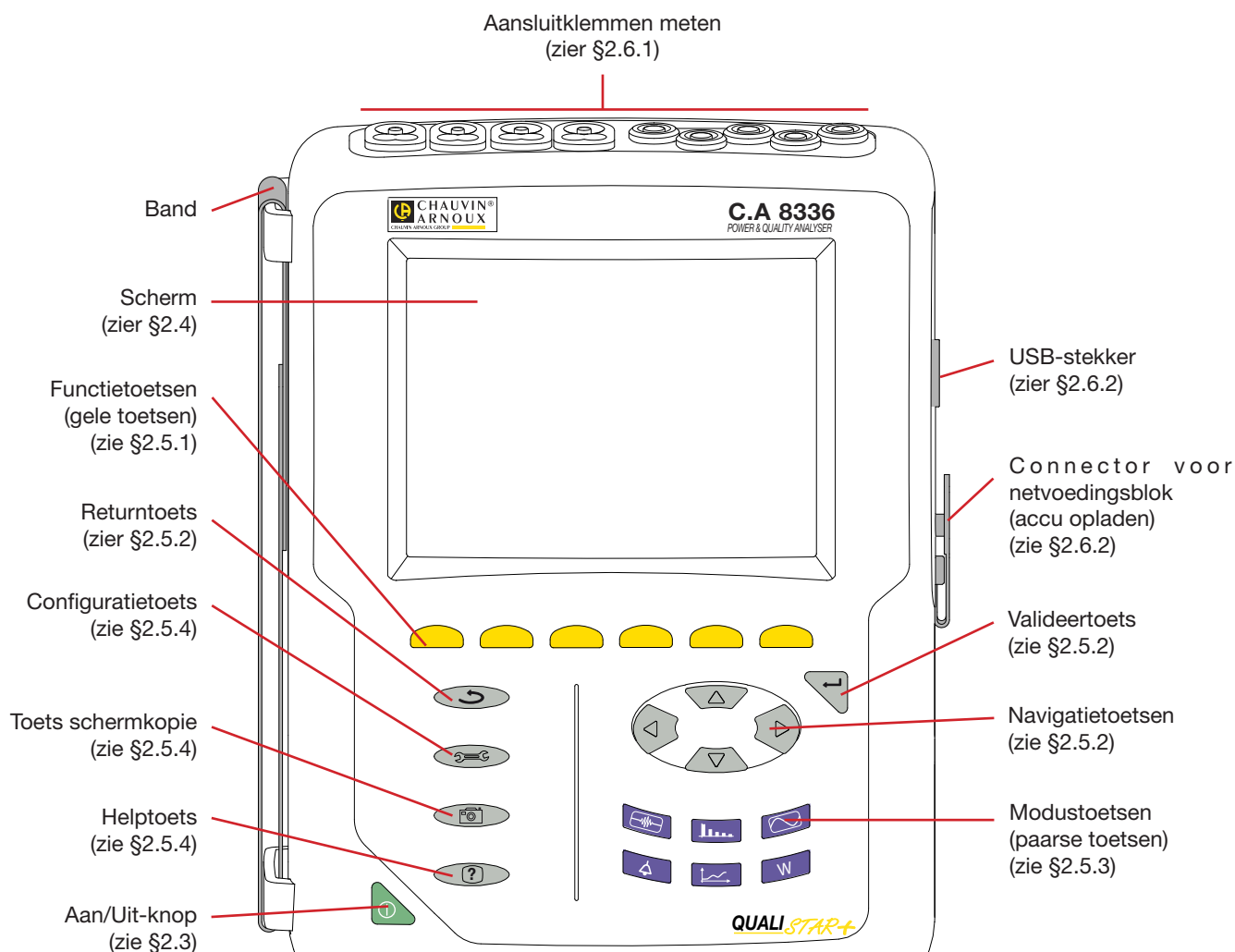
Figuur 1 : overzicht van de Qualistar+
