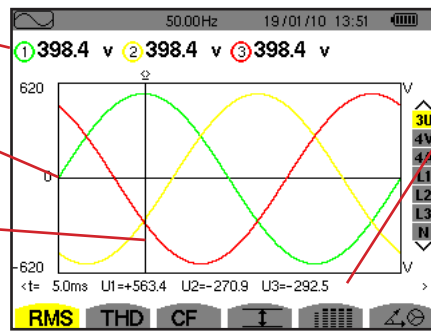
Figuur 63 : het beeldscherm RMS in 3U
