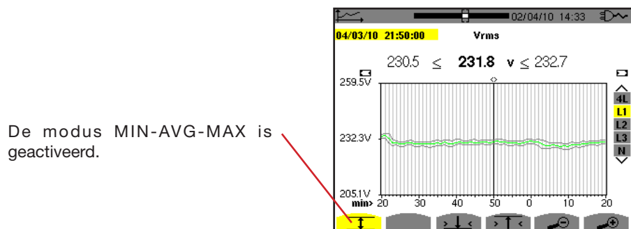
Figuur 96: Vrms (L1) met MIN-AVG-MAX
