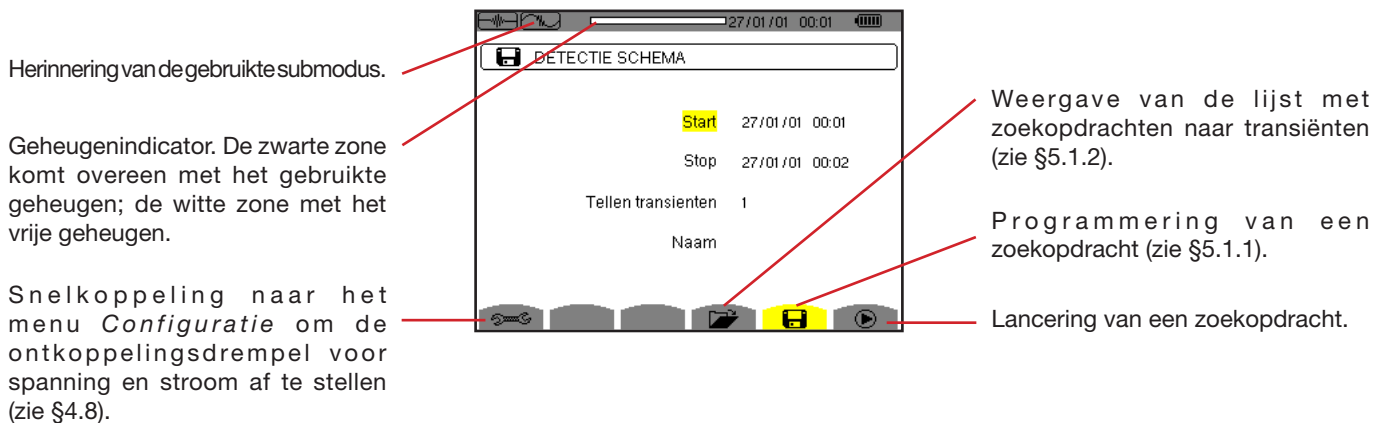
Figuur 38 : het scherm Programmering van een zoekopdracht in de transiëntmodus
