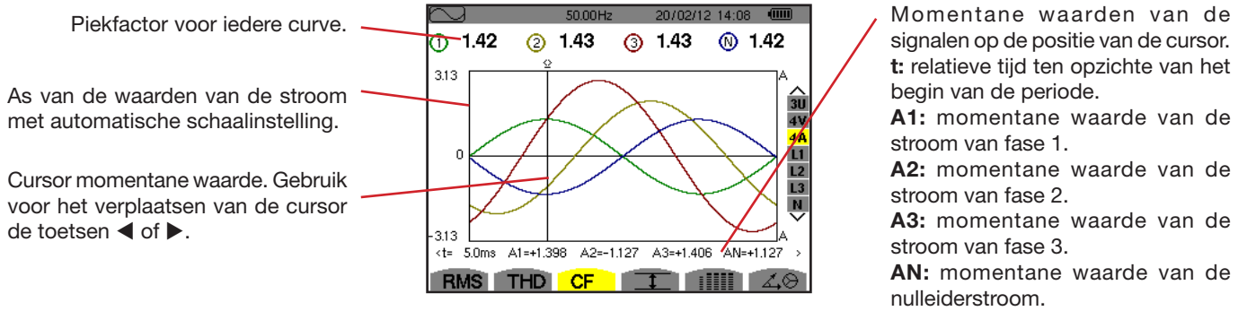
Figuur 72: het beeldscherm CF in 4A
