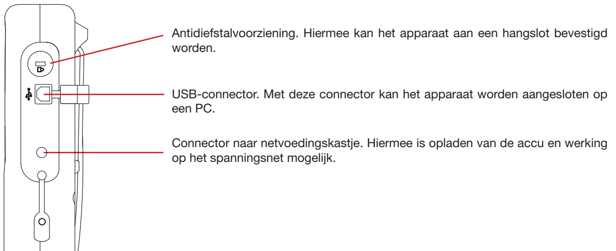
Figuur 4 : de zijconnectoren
