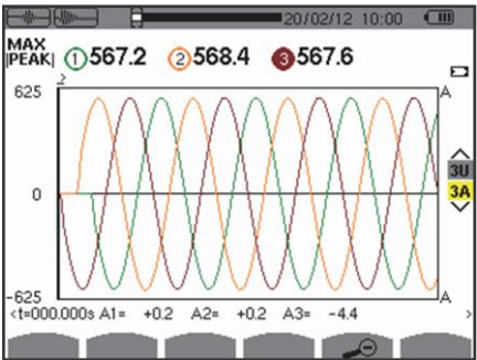
图49：三相三线连接的3A 峰值显示页面
