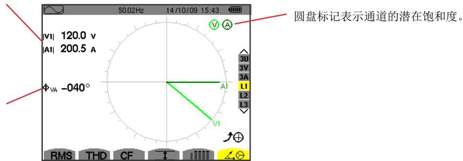
图82: L1 菲涅尔图显示页面
