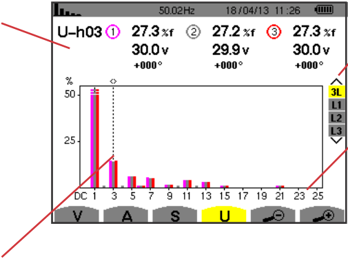
图58: 3L线电压谐波显示举例
