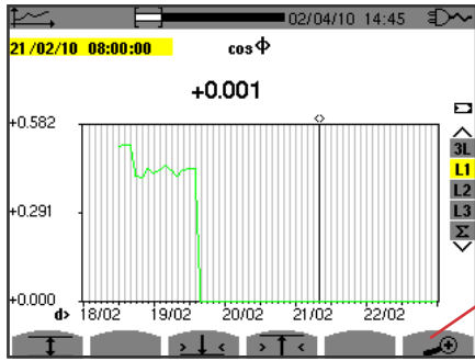
图95: 对于含中性线连接的三相不包含MIN-AVG-MAX的 \cos \sqrt{L1} 完整值读取/计算。
