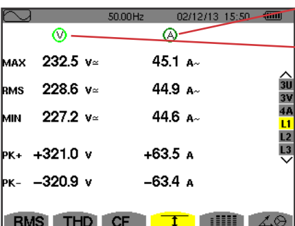
图66: L1 最大-最小显示页面
