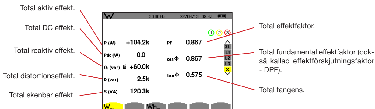
Figur 115: Skärm med totala effekterna och associerade enheter i \Sigma
