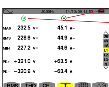
Figur 76: Visning av Max-Min värden i L1 läge
