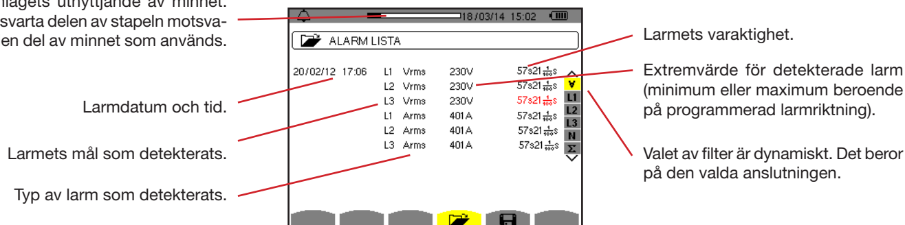
Figur 87: Skärm med larmlista
