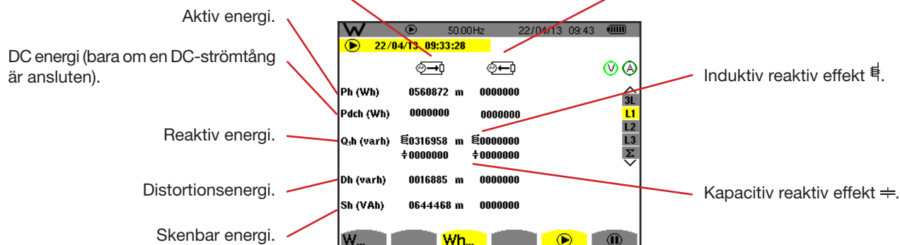
Figur 114: Skärm med förbrukad och genererad energi i L1
