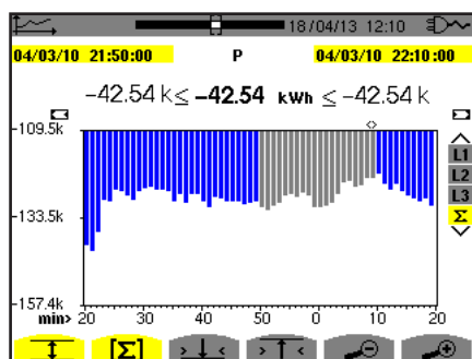
Figure 102 : Ph ( \Sigma ) avec MIN-AVG-MAX
