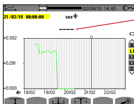
Figure 106 : cos Φ (L1) arrêt prématuré du chargement/calcul des valeurs.
