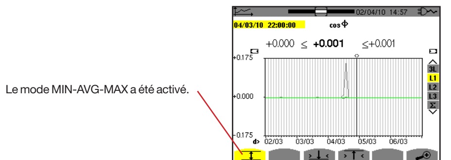
Figure 104 : \cos \Phi (L1) avec MIN-AVG-MAX
