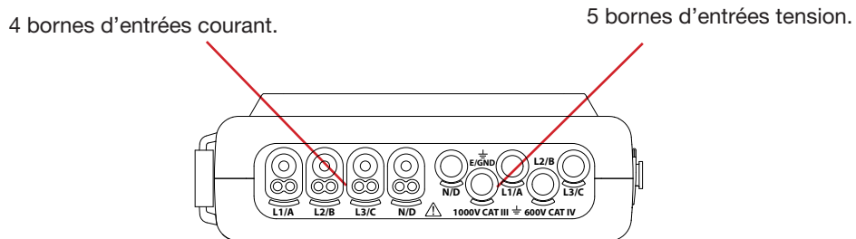
Figure 3 : les bornes de branchement
