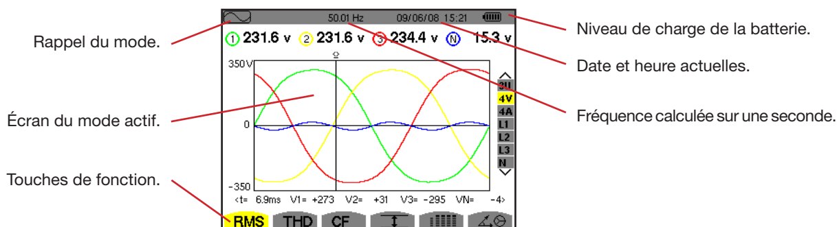
Figure 2 : exemple d'un écran de visualisation
