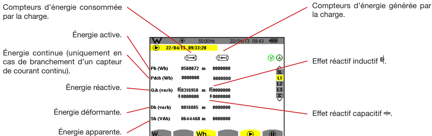
Figure 114 : l'écran d'affichage énergies consommées et générées en L1
