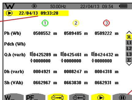
Figure 117 : l'écran de démarrage du comptage d'énergie en Wh
