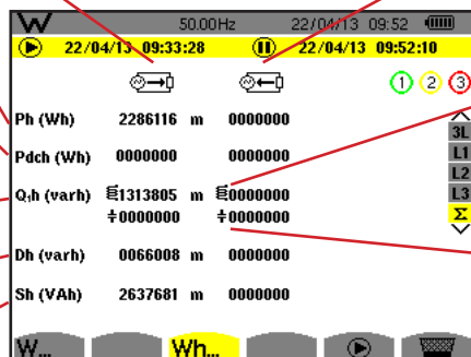
Figure 116 : l'écran d'affichage des énergies consommées et générées totales en \Sigma
