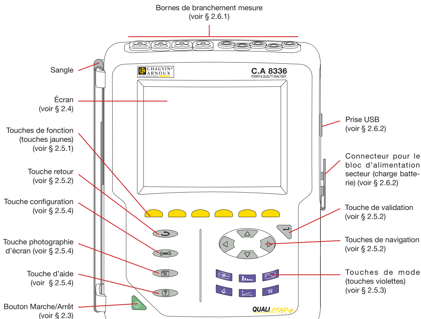
Figure 1 : vue générale du Qualistar+
