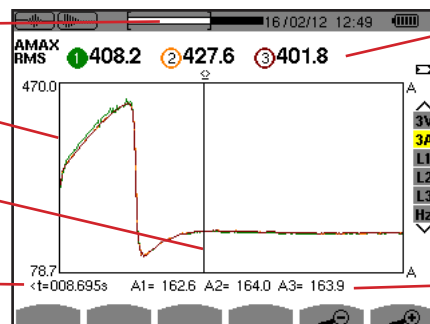
Figure 44 : l'écran d'affichage RMS en 3A pour un branchement triphasé avec neutre
