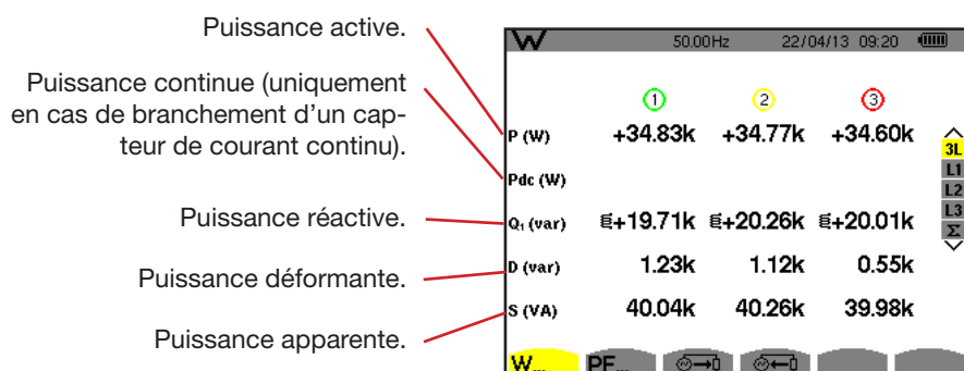
Figure 109 : l'écran des puissances en 3L.
