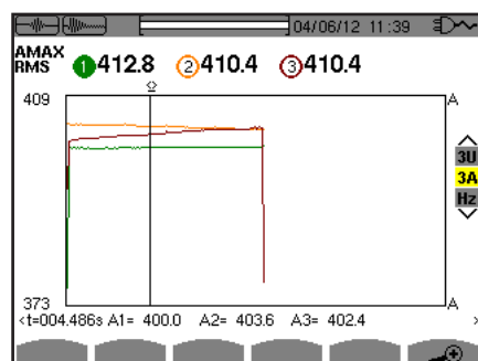
Figure 45 : l'écran d'affichage RMS en 3A pour un branchement triphasé sans neutre
