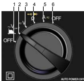
Figure 1 : le commutateur
