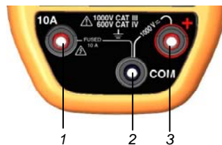
Figura 4 : los terminales
