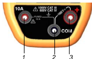
Figura 4 : i morsetti
