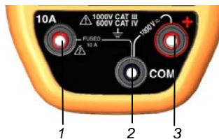
Figure 4 : les bornes
