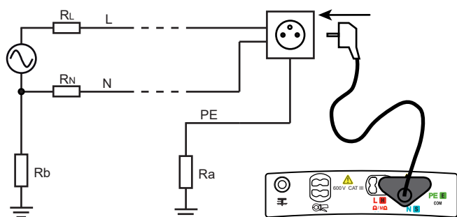
TT-laitteiston tapaus
