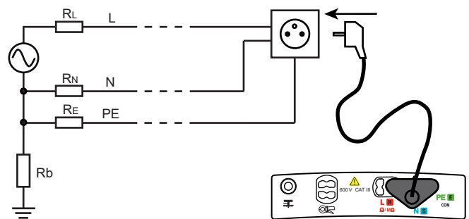
TN-laitteiston tapaus
