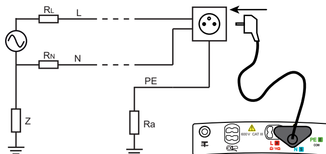
IT-laitteiston tapaus
