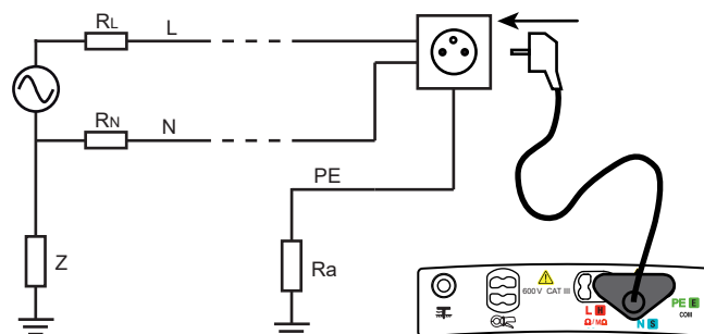
Geval van een IT installatie
