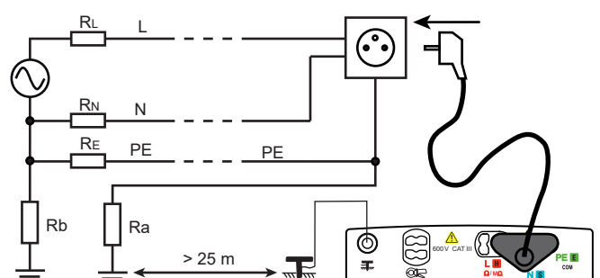
Vid TN-installation
