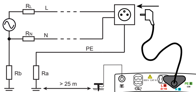
Vid TT-installationer.
