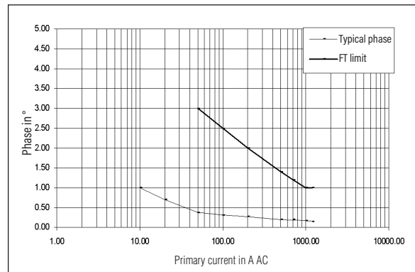
Phase shift
