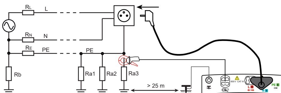
Případ soustavy typu TN
