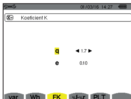
Obrázek 22: Nabídka pro volbu součinitelů pro výpočet činitele K
