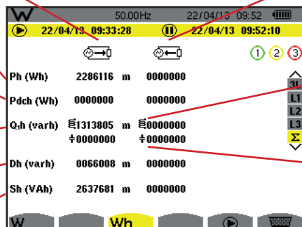
Obrázek 116: Obrazovka celkových energií spotřebovaných a generovaných v \Sigma
