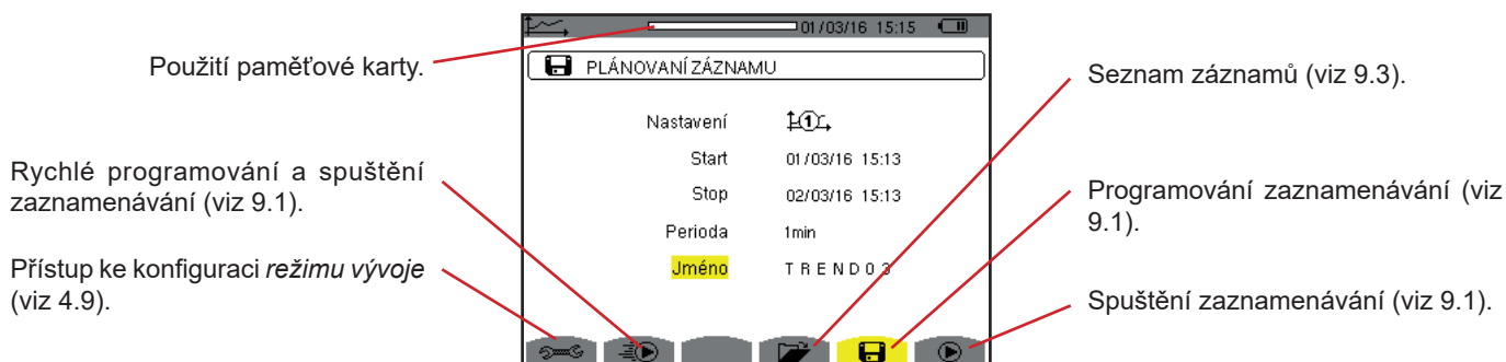
Obrázek 88: Obrazovka režimu vývoje
