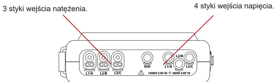
Rysunek 11 : Styki podłączeniowe
