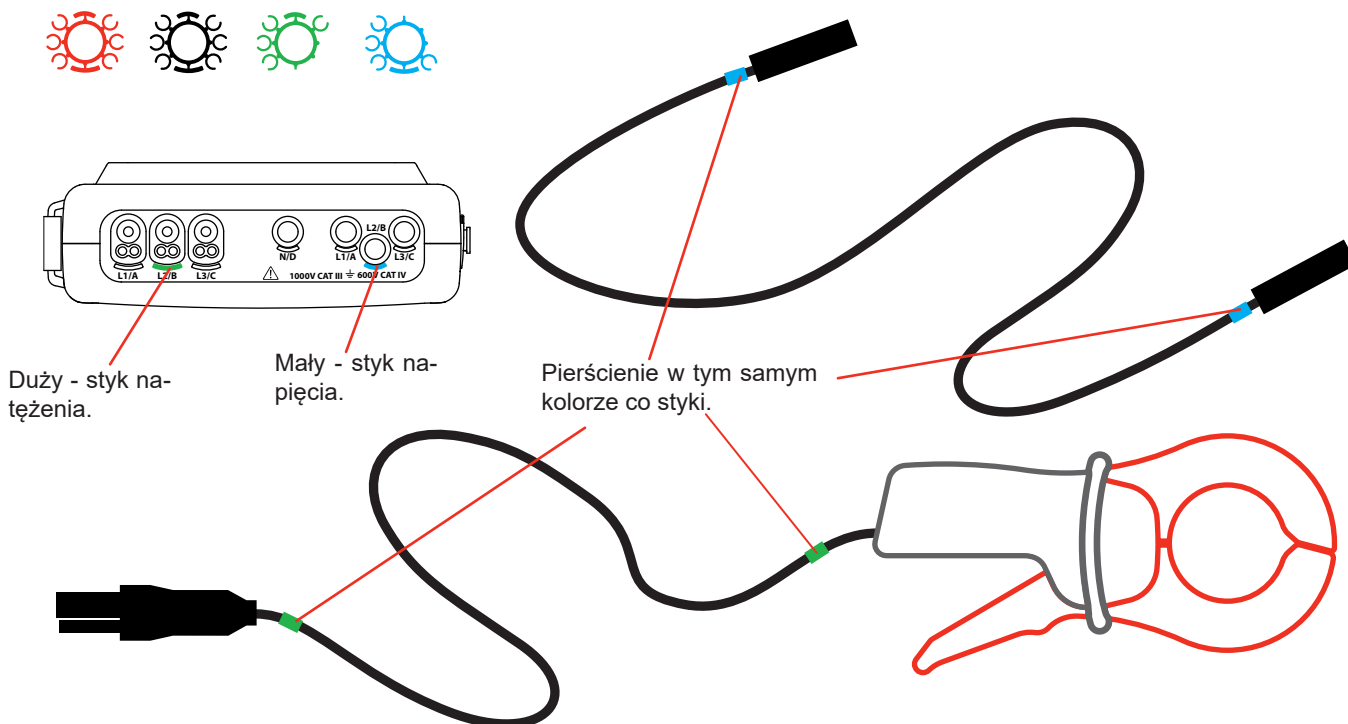
Rysunek 10 : Identyfikacja przewodów i styków
