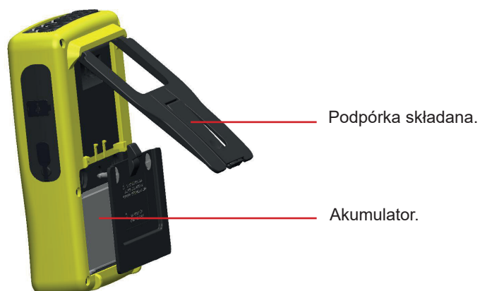
Rysunek 5: podpórka i pokrywa zasobnika akumulatora
