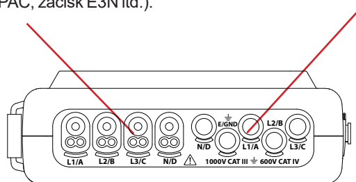
Rysunek 3: styki podłączeniowe
