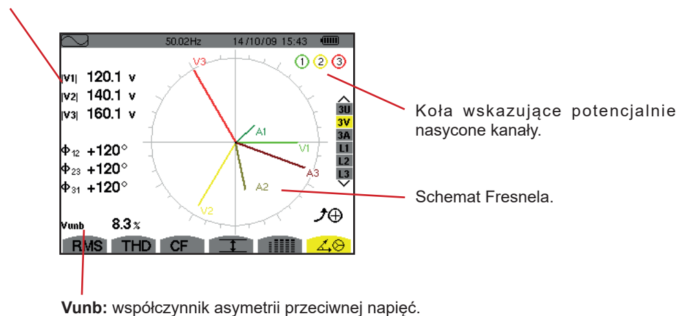
Rysunek 82: ekran wyświetlania wykresu Fresnela w 3V
