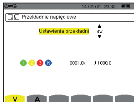
Rysunek 27: ekran Współczynników napięcia w menu Czujniki i współczynniki w przypadku montażu z zerem
