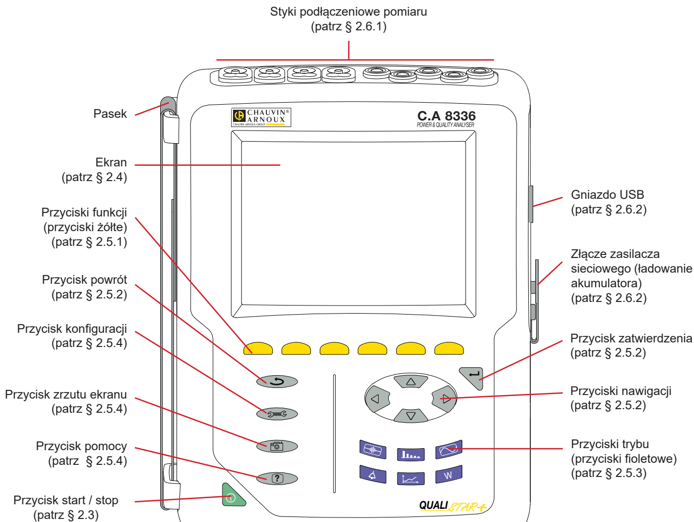
Rysunek 1: widok ogólny Qualistar+
