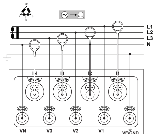
4.1.5.2. Sieć trójfazową z 4 przewodami \Delta otwartą:
