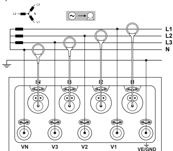
4.1.4.2. Sieć trójfazowa z 4 przewodami Y symetrycz-
