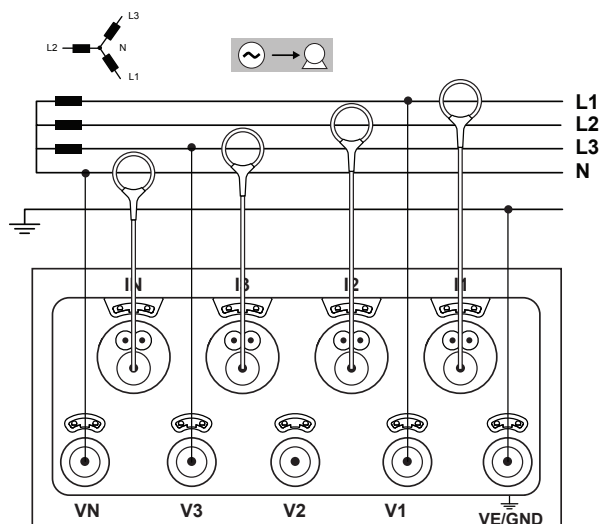
4.1.5. SIEĆ TRÓJFAZOWA Z 4 PRZEWODAMI \Delta
