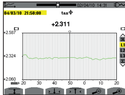
Figuur 85 : \tan \Phi (L1) zonder MIN-AVG-MAX voor een driefasen aansluiting met nulleider
