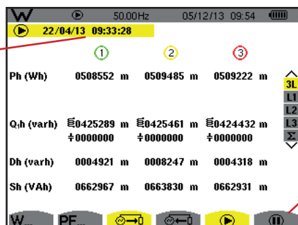
Figuur 105 : Het scherm van het opstarten van de energietelling in Wh
