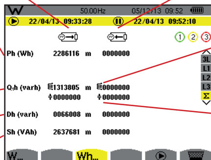
Figuur 104 : Het beeldscherm van de totaal verbruikte en gegenereerde energiewaarden in Σ
