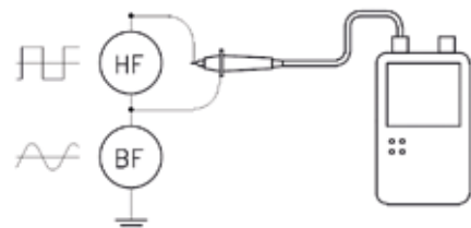
Correct : faible courant de masse
