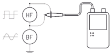
Incorrecte : fort courant de masse
