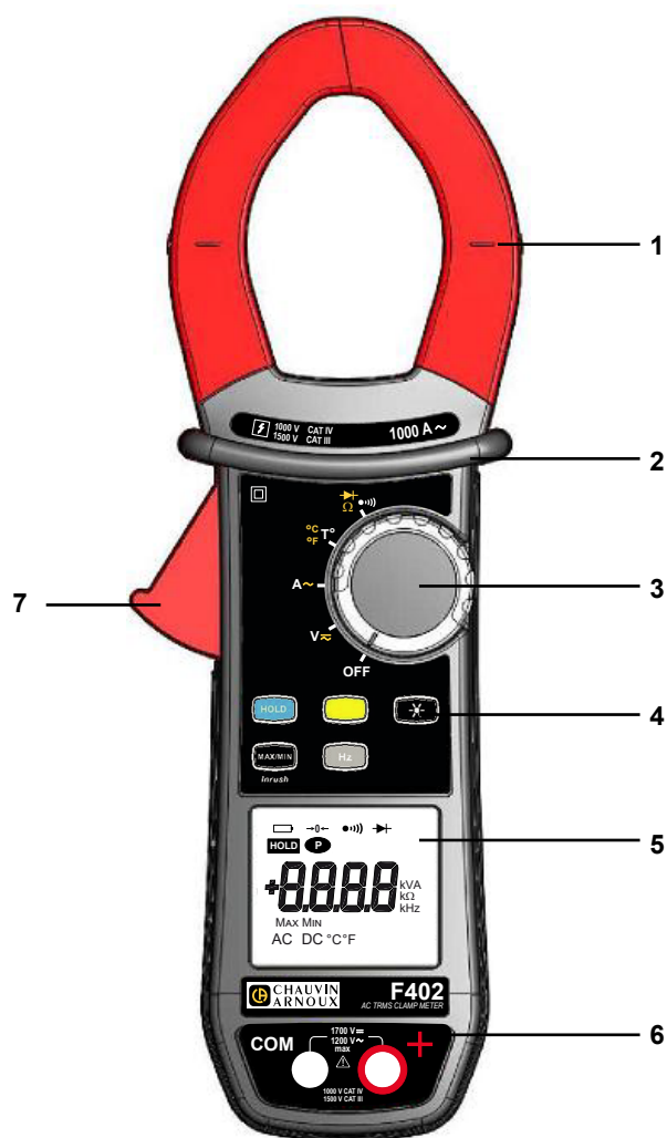
Kuva 1: F402-monitoimipihtimittari
