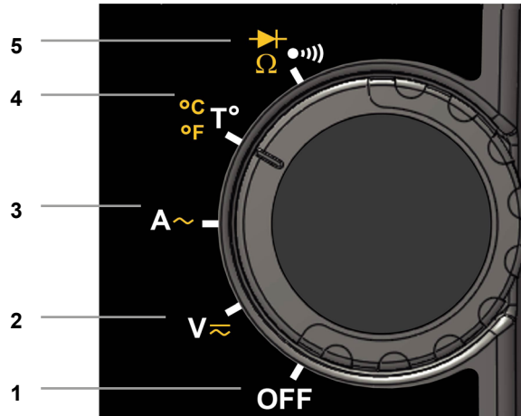
Kuva 2: kiertytkin
