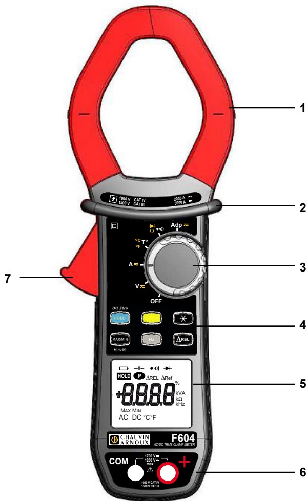
Figura 1: Cleștele multimetru F604
