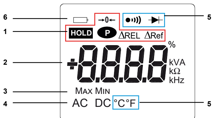
Figura 4: Afişajul
