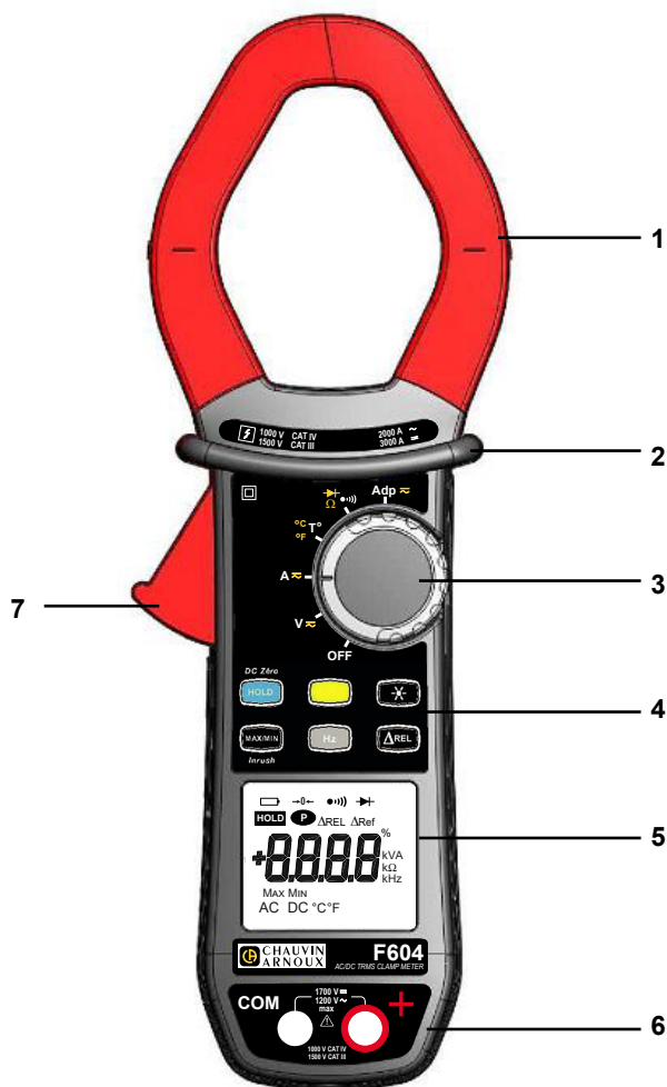
Figuur 1 : de multimeter tang F604
