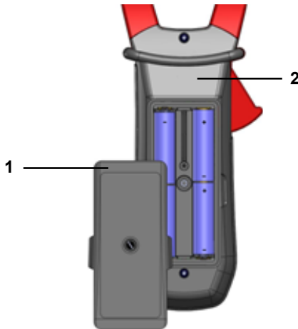
Figuur 6: De klep van het batterijvakje
