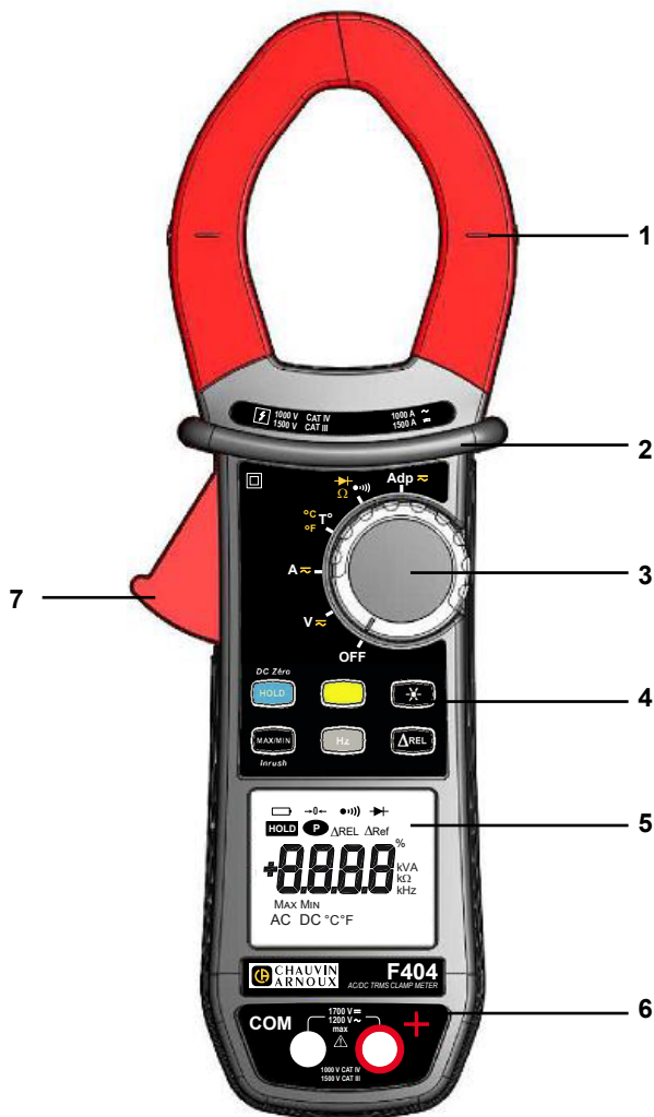
Figuur 1 : de multimetertang F404
